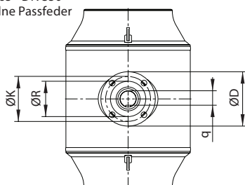
DN 65 - DN 350 Einzelne Passfeder
