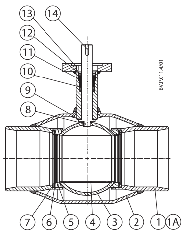
DN 65–200 mit Getriebeflansch
