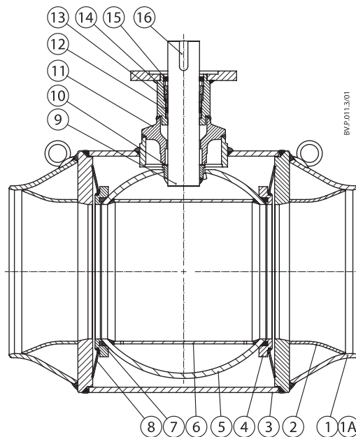
DN 250–600 mit Getriebeflansch
